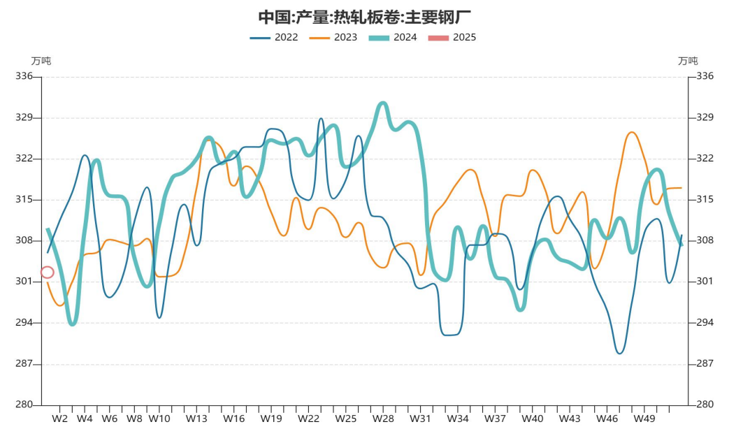
图11、热卷产量
