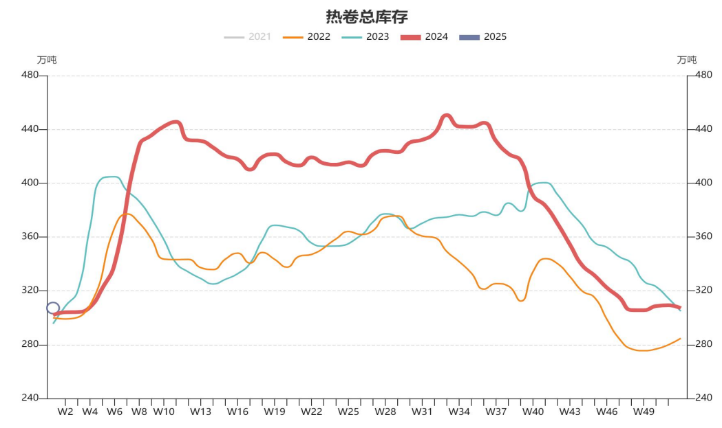
图13、热卷总库存
