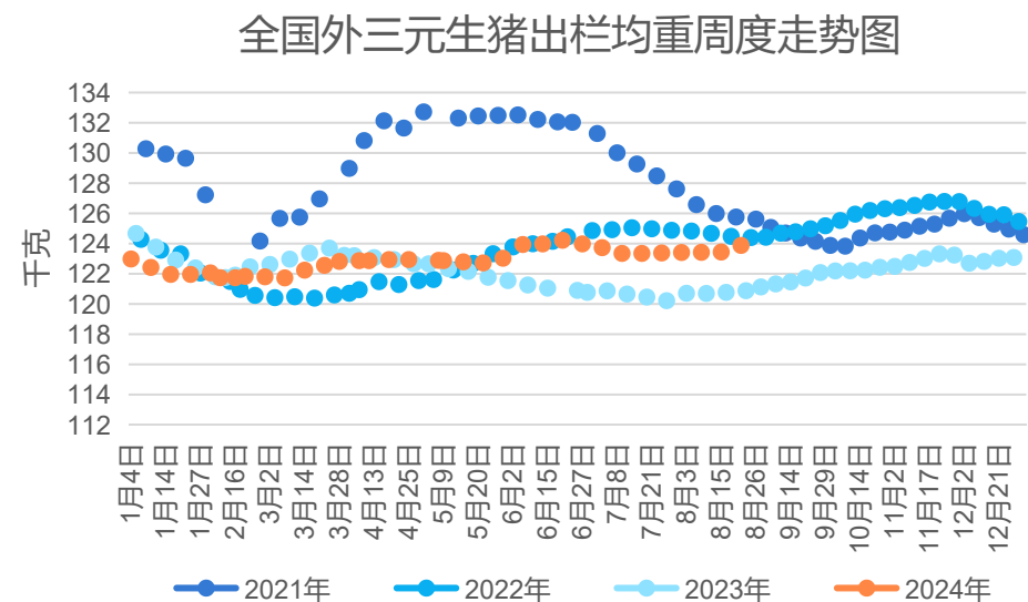
图12、出栏均重
