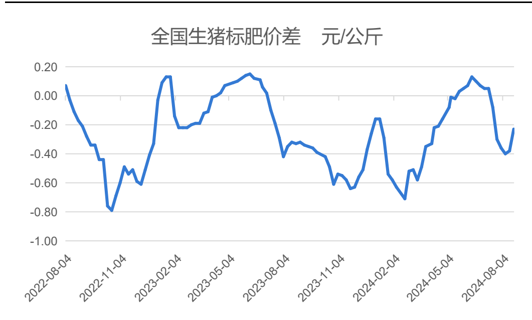
图18、标肥价差
