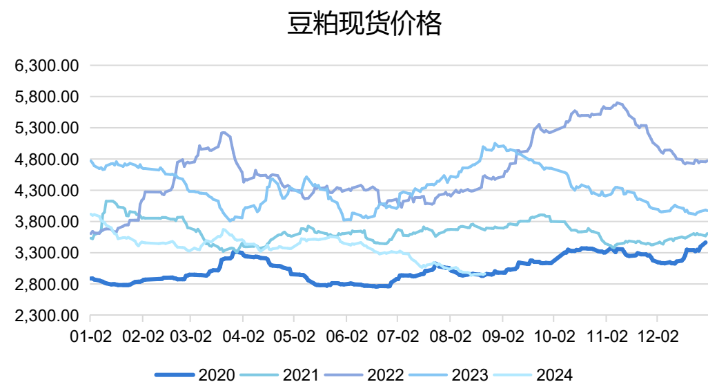
图19、豆粕价格
