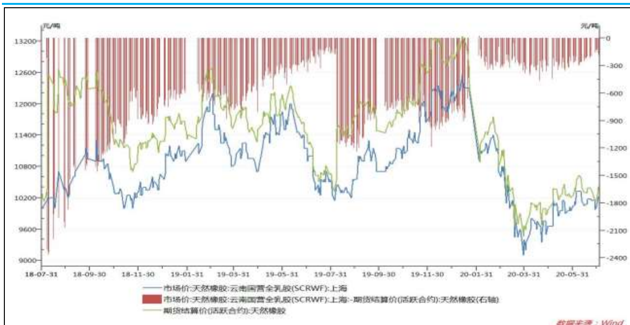
图6 沪胶基差
