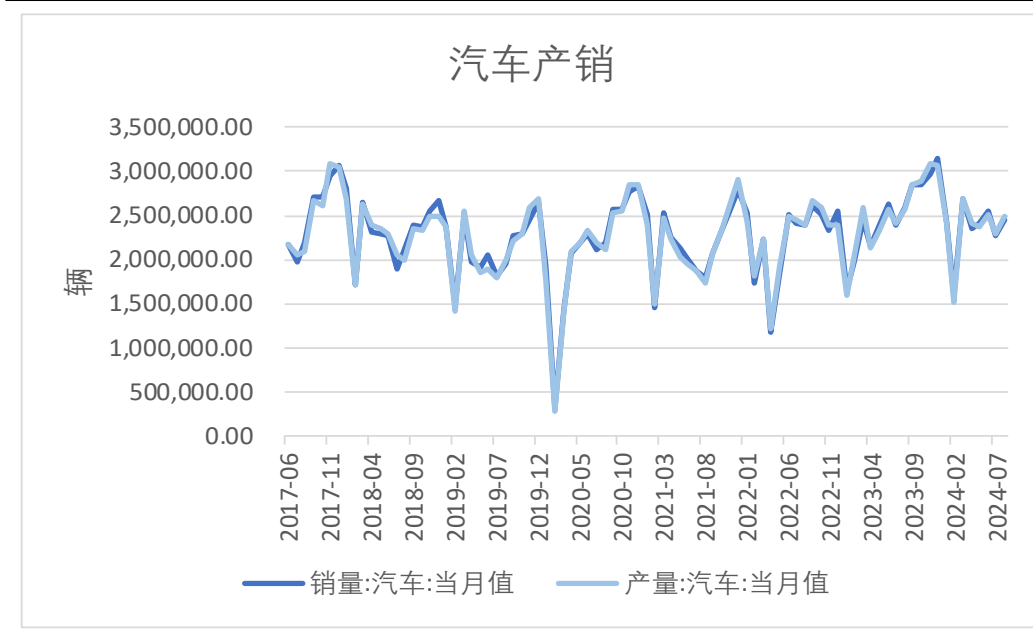
图15、汽车产销
