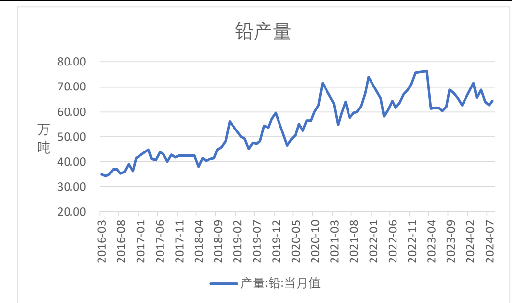
图13、铅产量
